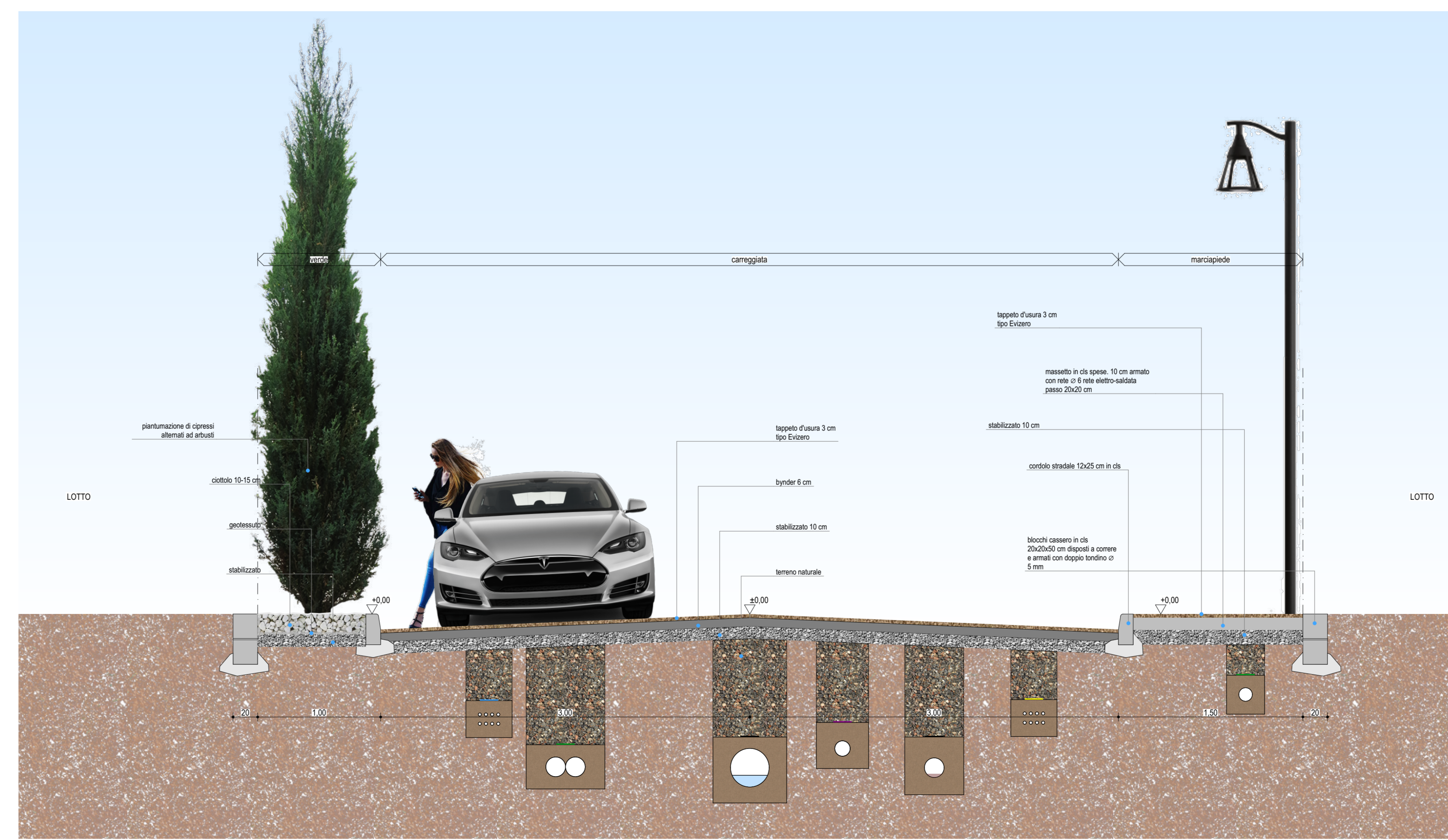
Det-01 Sezioni stradali 1:25
